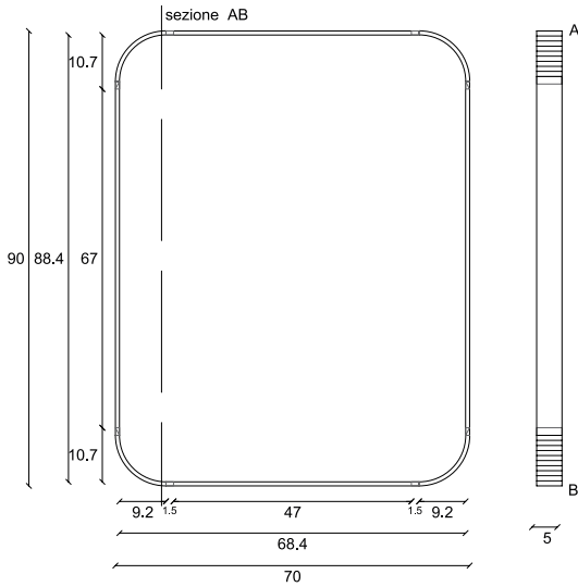
Greek Mirror DIM. 70L x 90H Cromo Nero Lucido Oro 0013790 0013791 0013792
