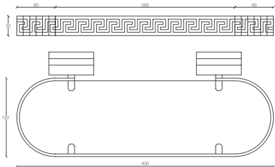
Greek Mensola Shelf DIM. 40L x 12H Cromo Nero Lucido Oro 0013998 0013999 0014000
