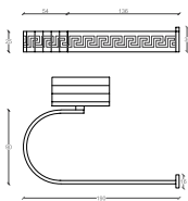
Greek Porta Rotolo Paper Holder DIM. 33L x 17H Cromo Nero Lucido Oro 0014004 0014005 0014006
