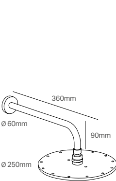
Soffione con braccio Shower head with arm
