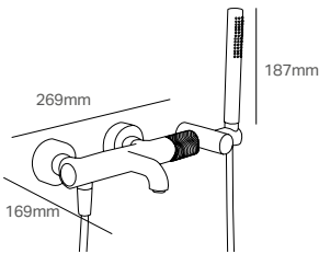
Miscelatore vasca esterno con set doccia Exposed bath mixer with shower set
