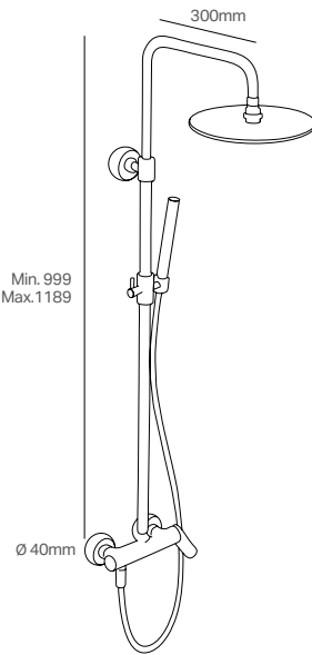
Miscelatore doccia esterno con colonna doccia soffione e doccetta Shower column with showerhead and shower set
